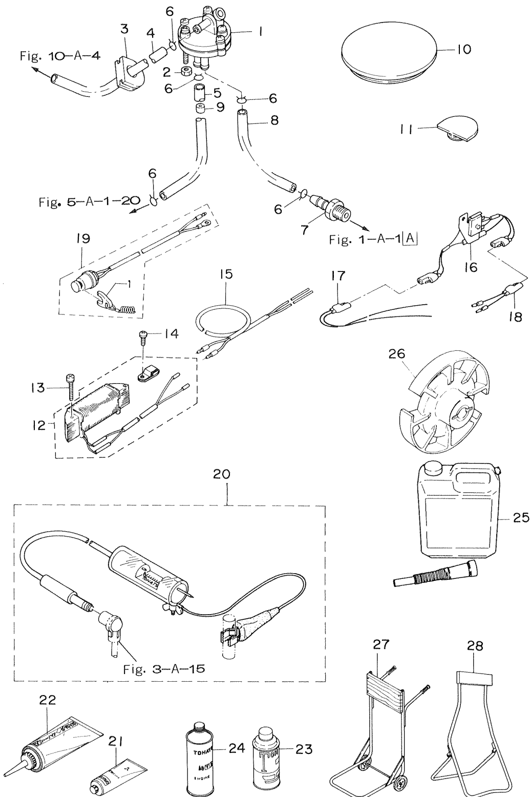
Fig. 12-A OPTIONAL PARTS(3)ACCESSORIES
