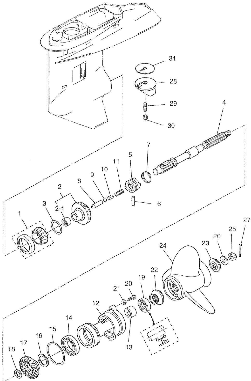
ギヤケース (プロペラシャフト) Fig. 2 GEAR CASE (PROPELLER SHAFT)
