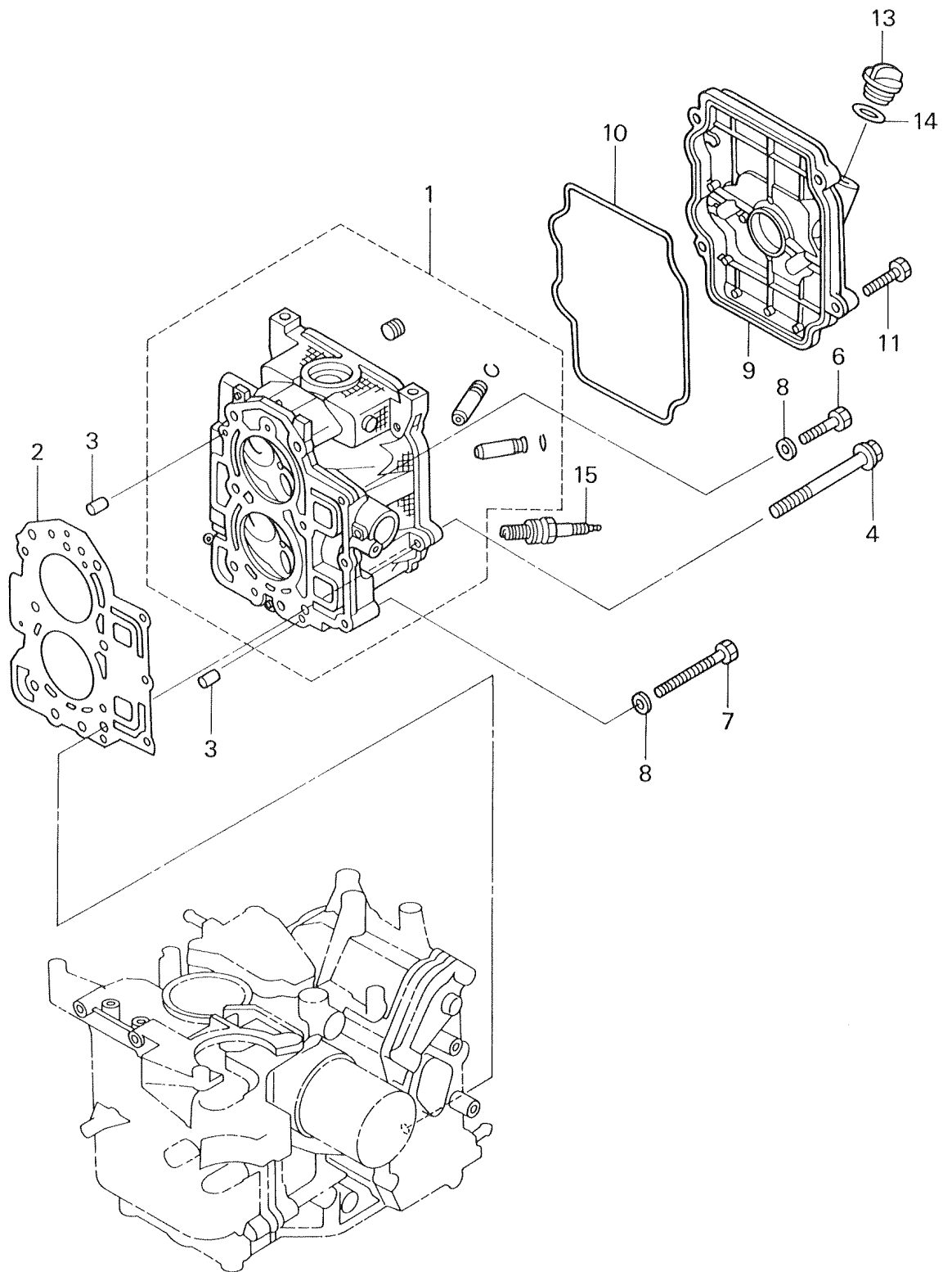
シリンダヘッド CYLINDER HEAD Fig. 1
