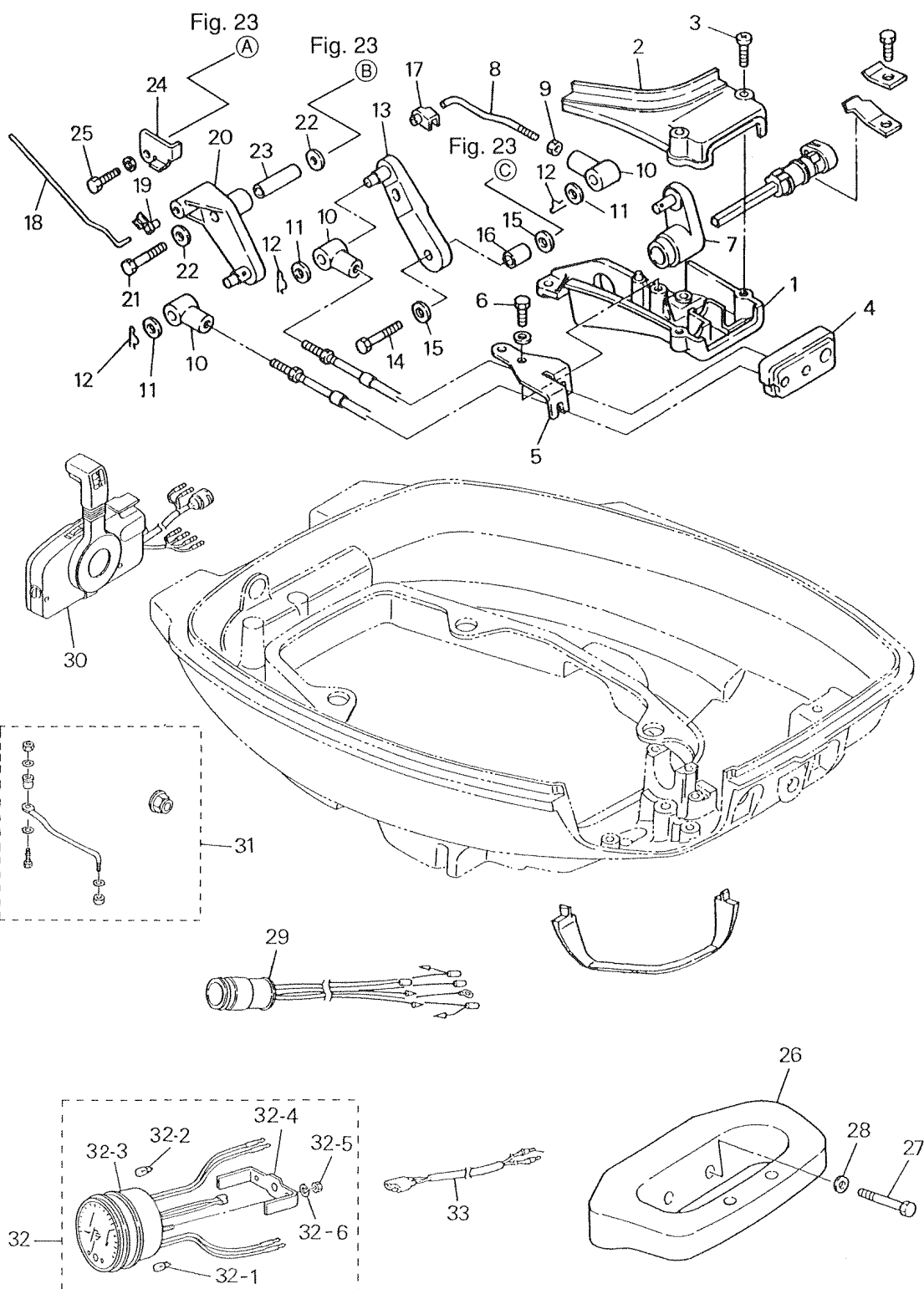
Fig. 17 シフト (EPモデル用) SHIFT (For EP)
