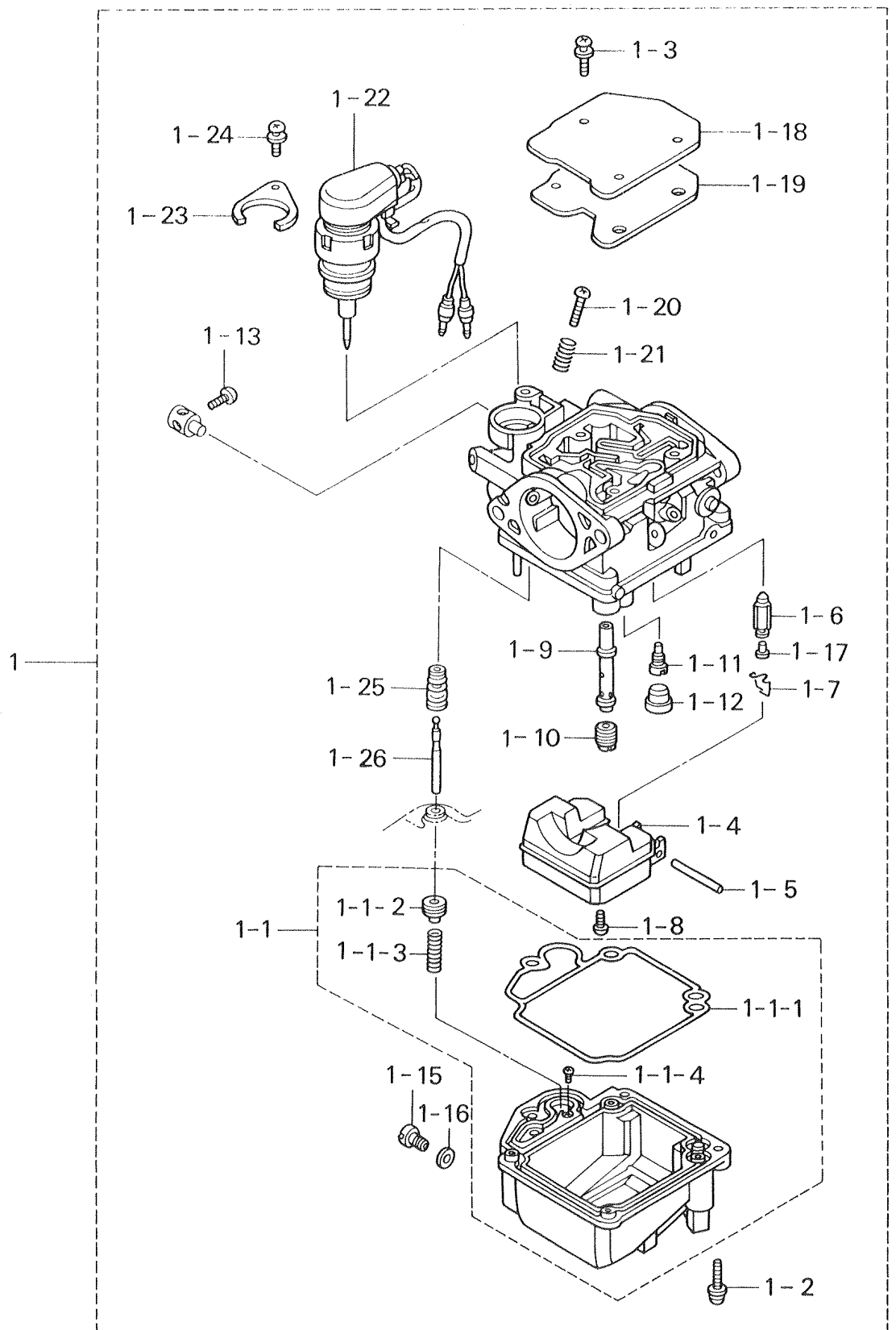
キャブレタ Fig. 5 CARBURETOR
