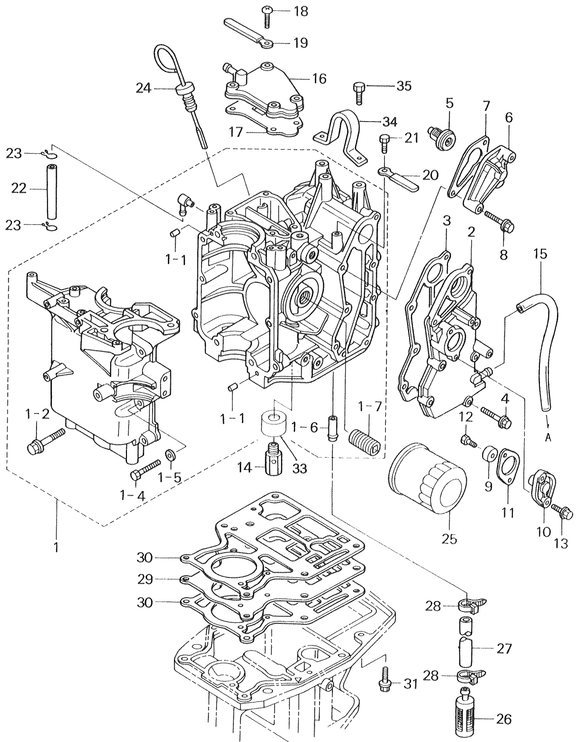
シリンダ CYLINDER Fig. 2
