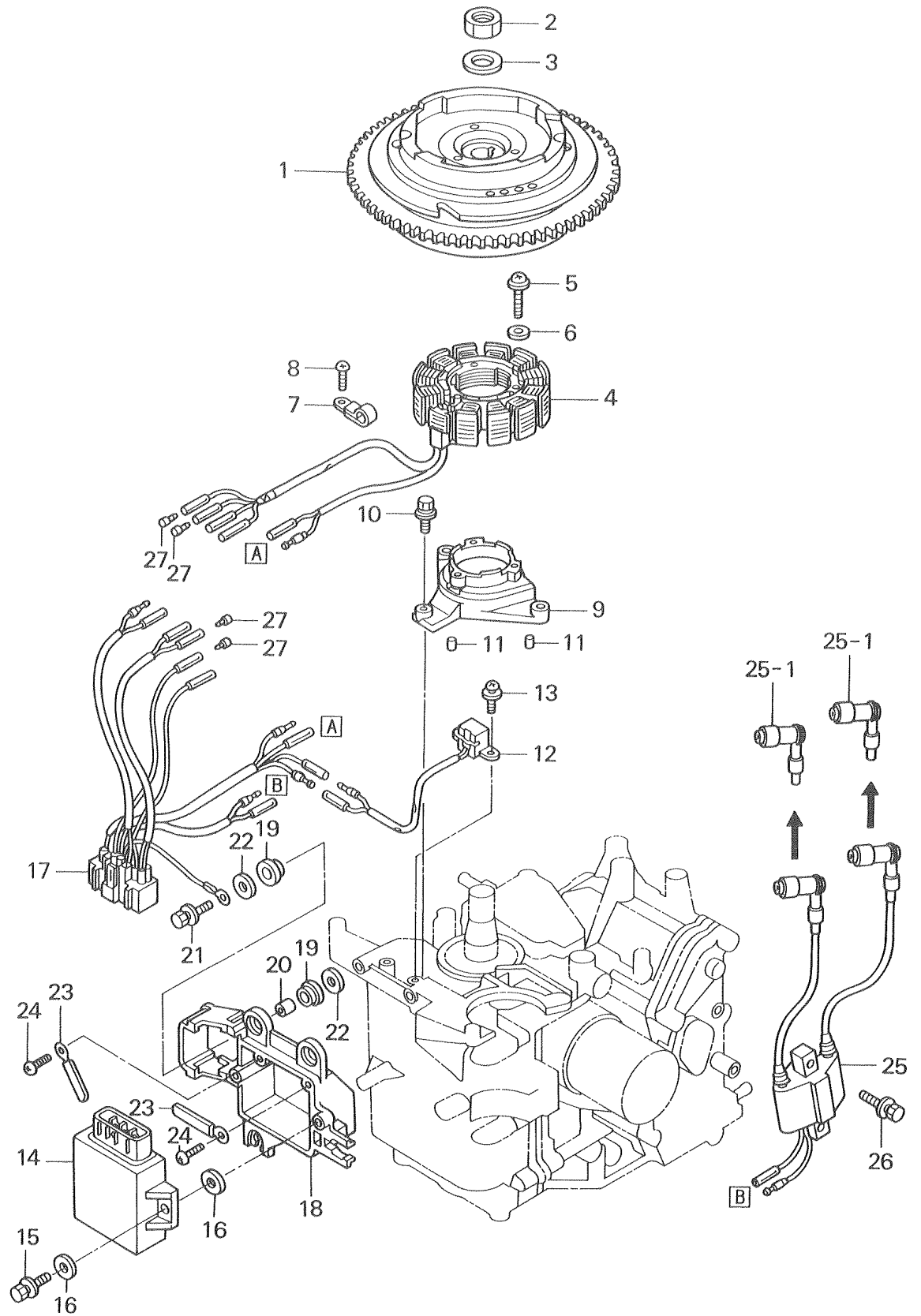
Fig. 8 マグネト MAGNETO
