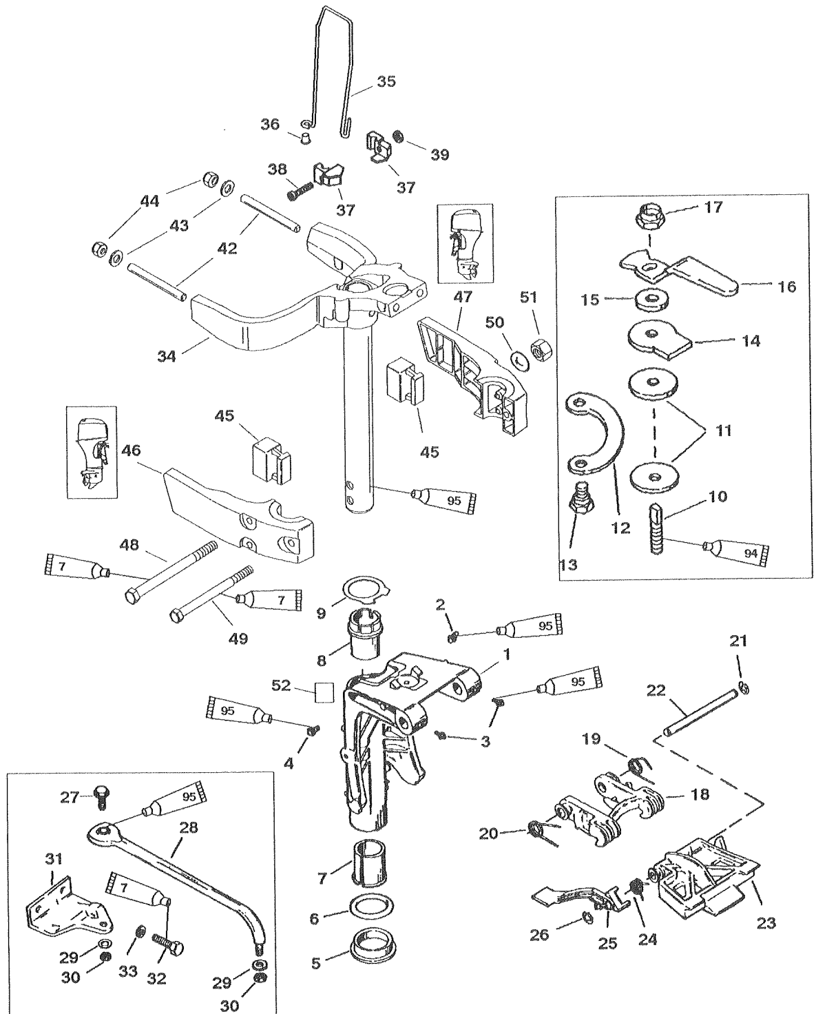
スウィベルブラケット Fig. 18 SWIVEL BRACKET
