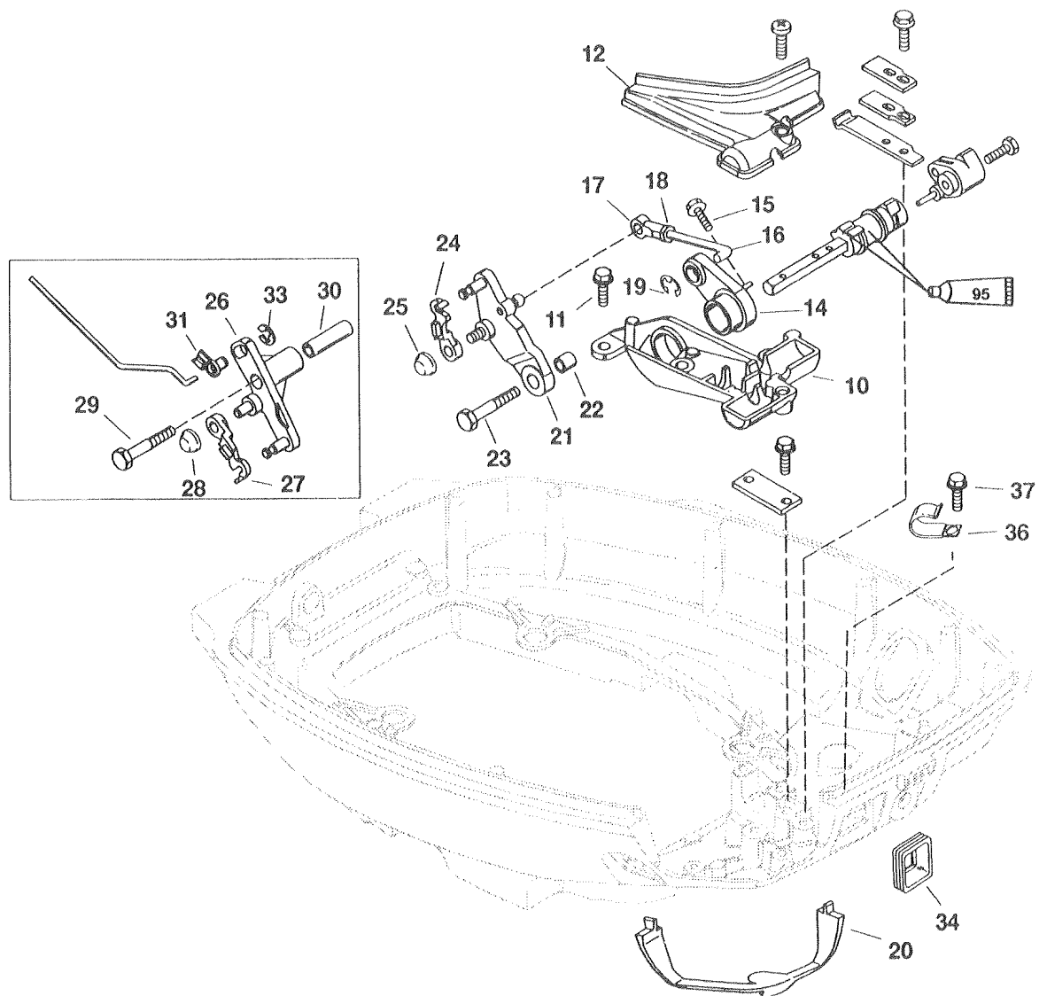
シフト (EPモデル用) Fig. 17 SHIFT (For EP)
