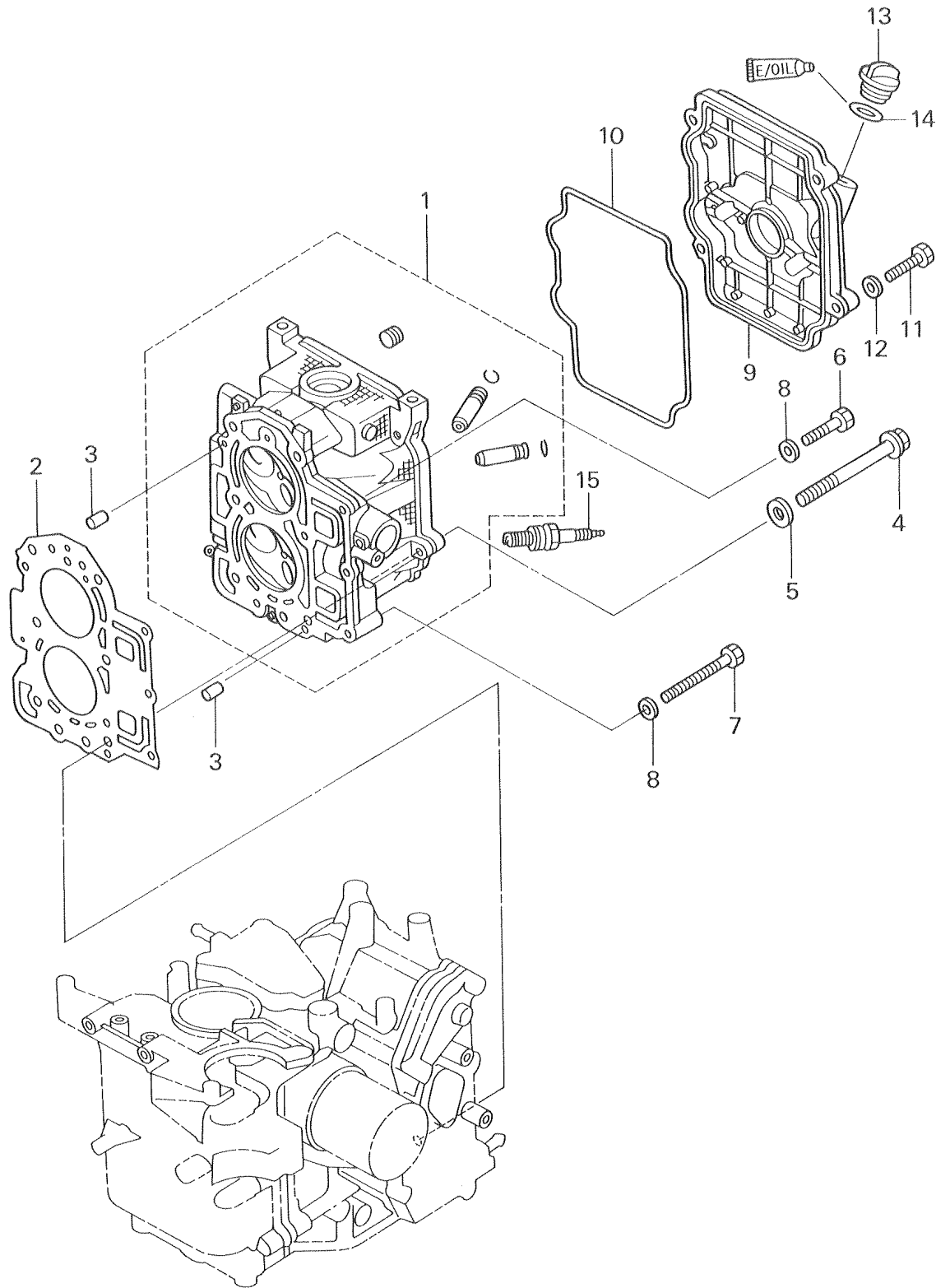
Fig. 1 シリンダヘッド CYLINDER HEAD
