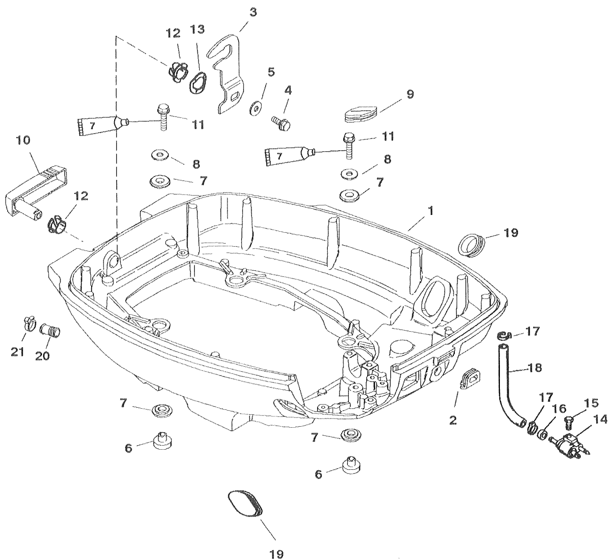
ボトムカウル&フュエルコネクタ Fig. 21 BOTTOM COWL & FUEL CONNECTOR
