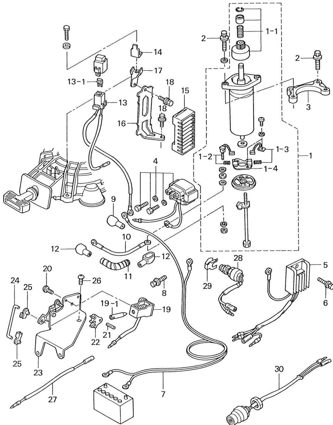
Fig. 9 エレクトリックパーツ ELECTRIC PARTS
