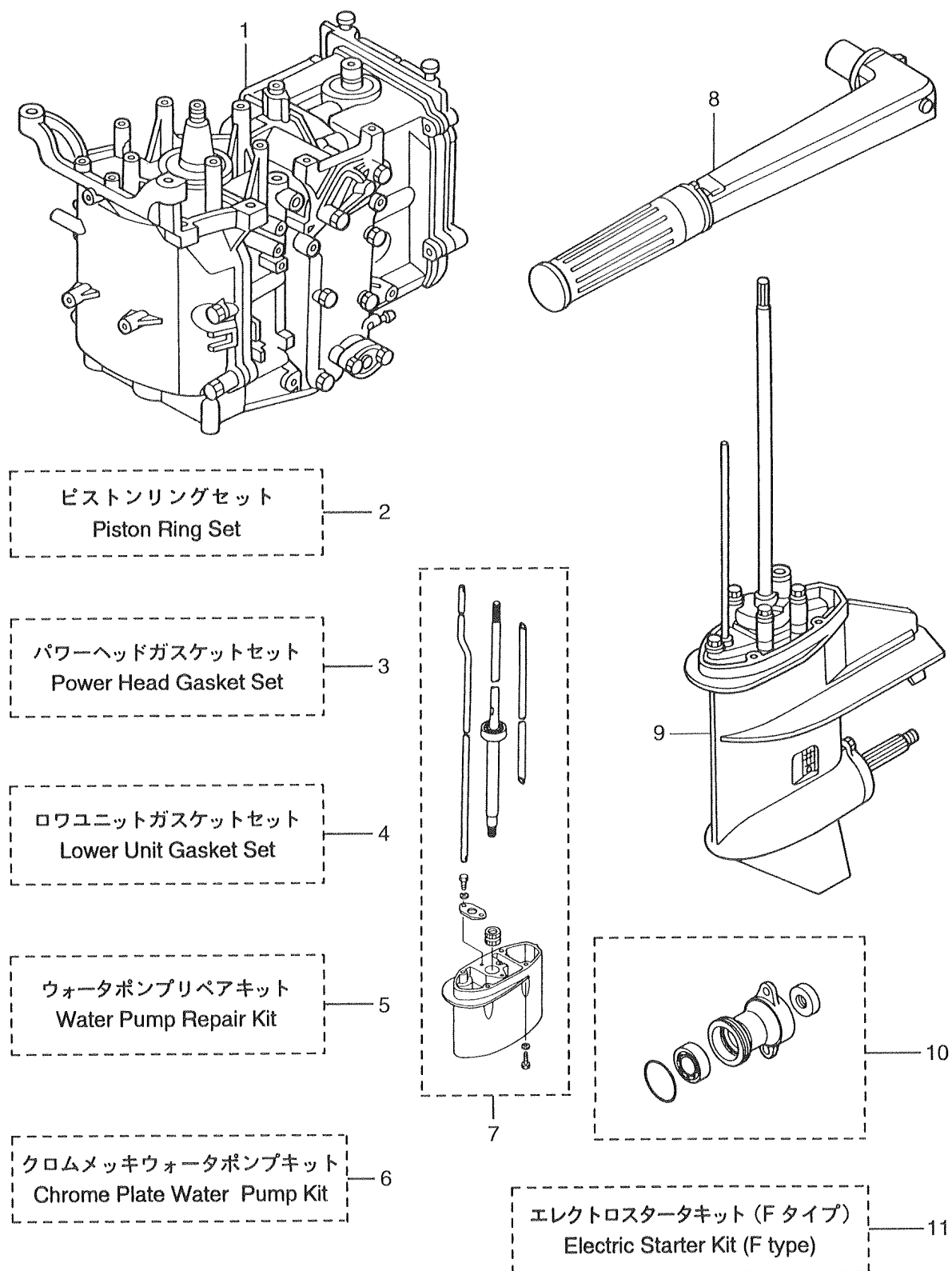
Fig. 20 アッセンブリ、キット ASSEMBLY, KIT
