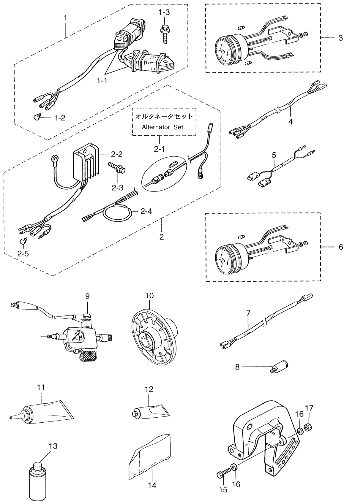
Fig. 21 オプショナルパーツ OPTIONAL PARTS
