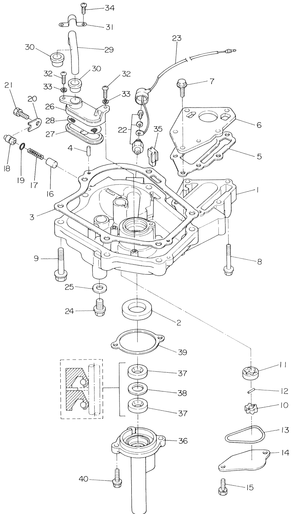
オイルパン Fig. 4 OIL PAN
