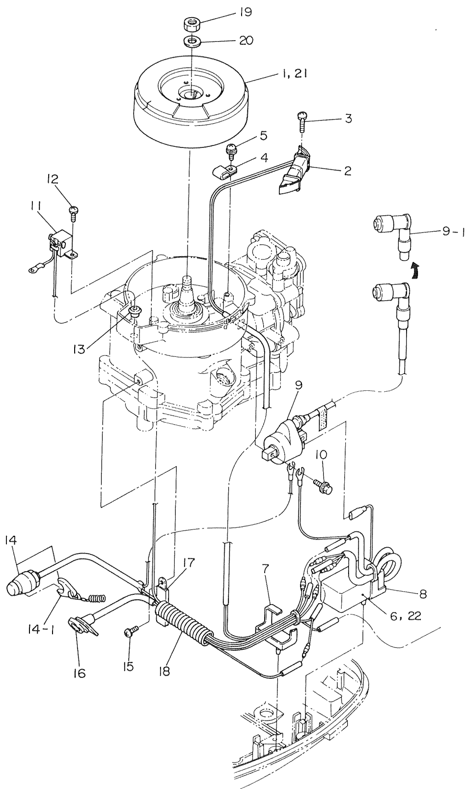
マグネト Fig. 6 MAGNETO
