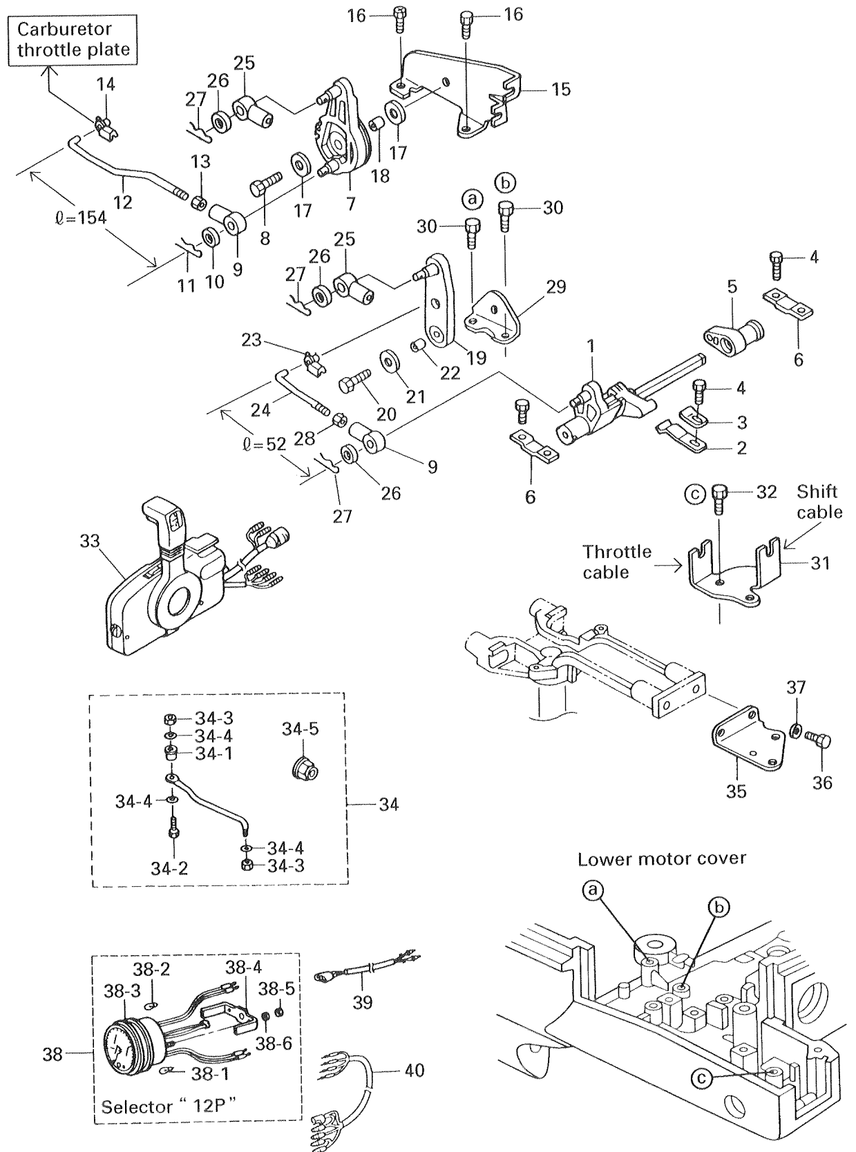
シフト SHIFT Fig. 17
