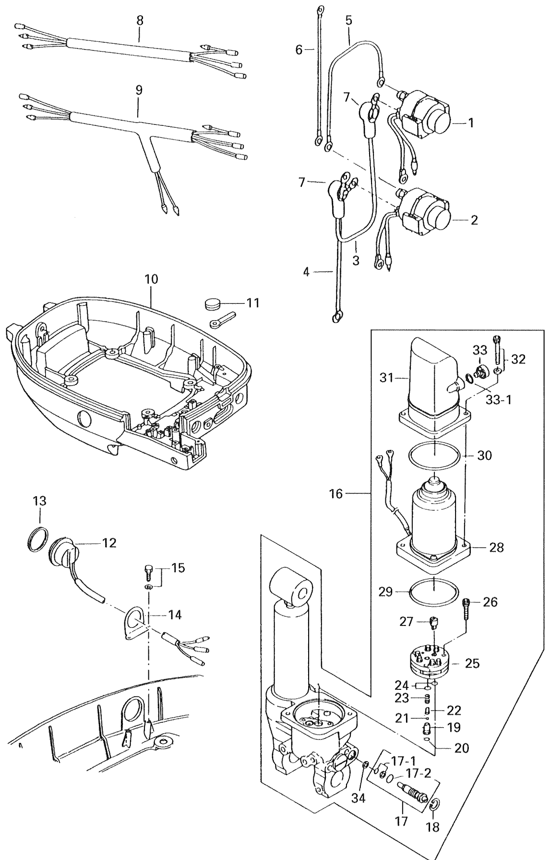
パワートリム&チルト・モータカバーロウ Fig. 21 POWER TRIM & TILT · MOTOR COVER LOWER
