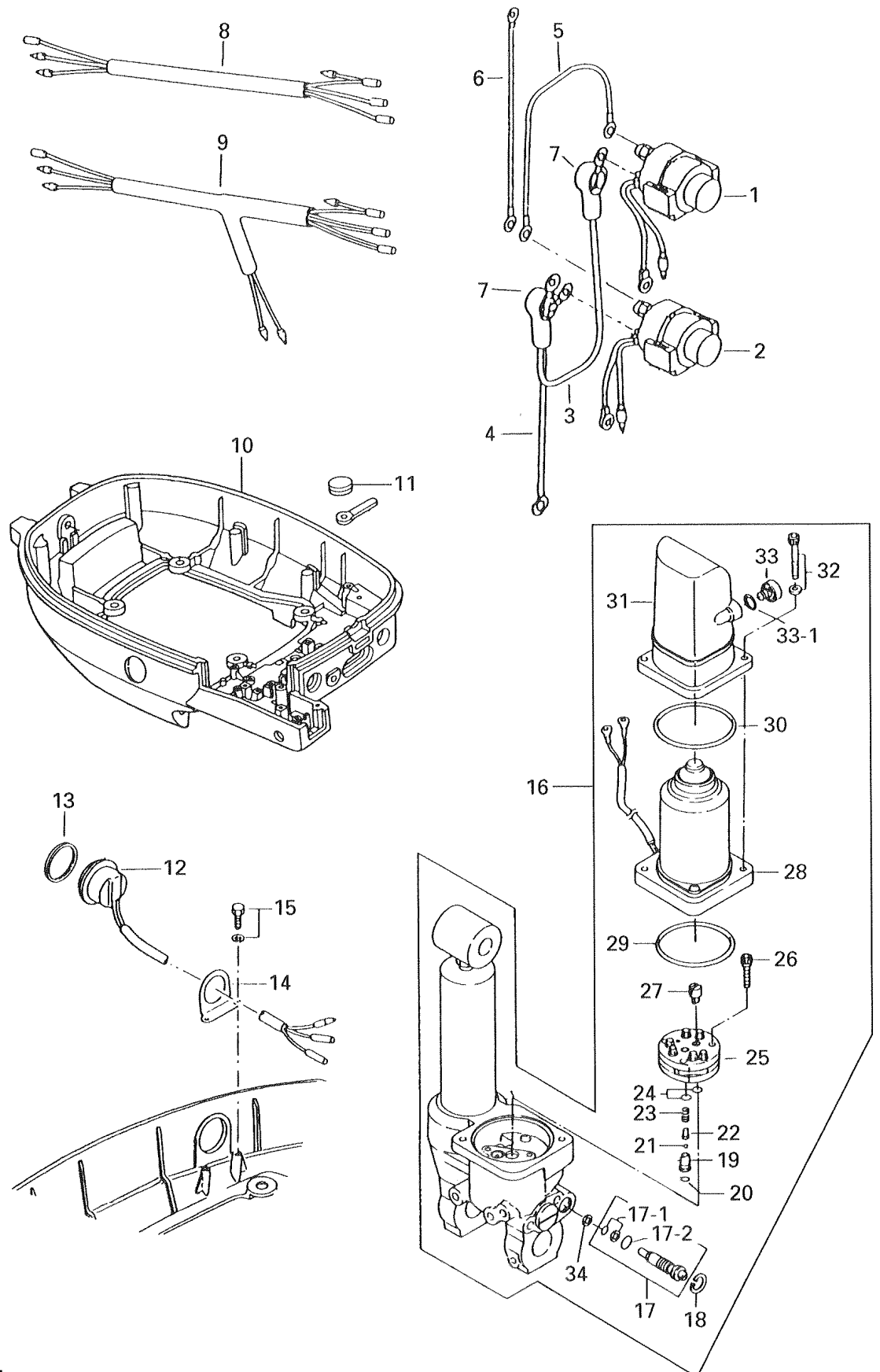
パワートリム&チルト・モータカバーロワ Fig. 21 POWER TRIM & TILT · MOTOR COVER LOWER
