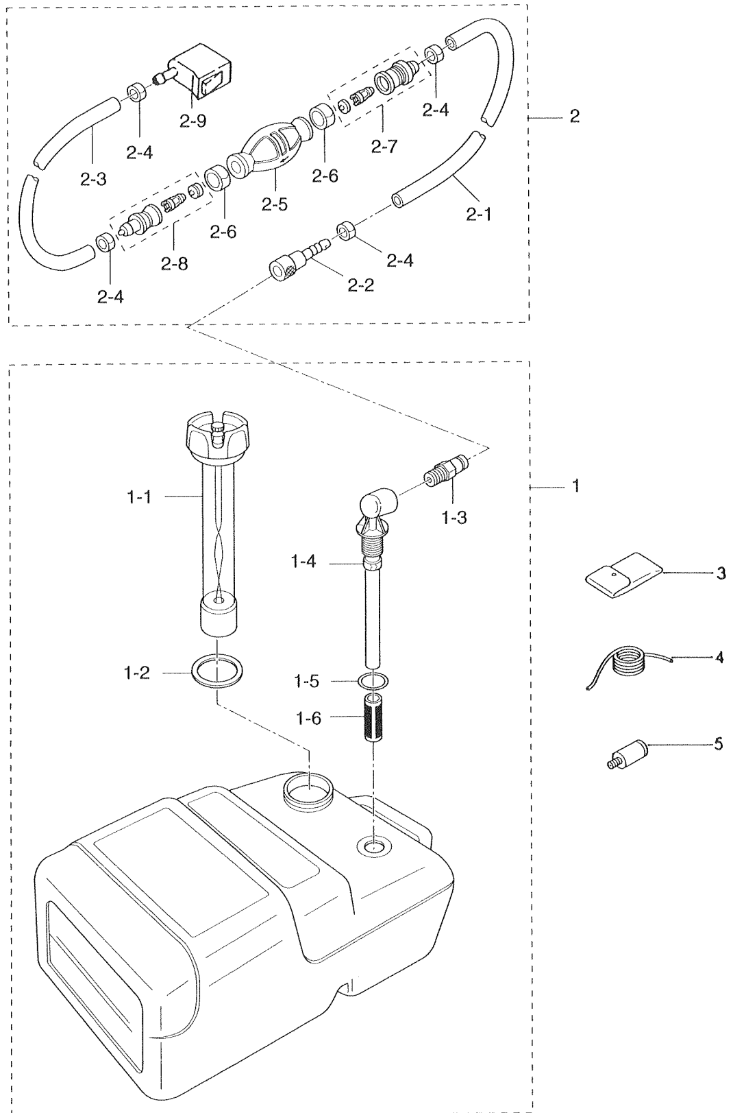
セパレートフュエルタンク Fig. 24 SEPARATE FUEL TANK
