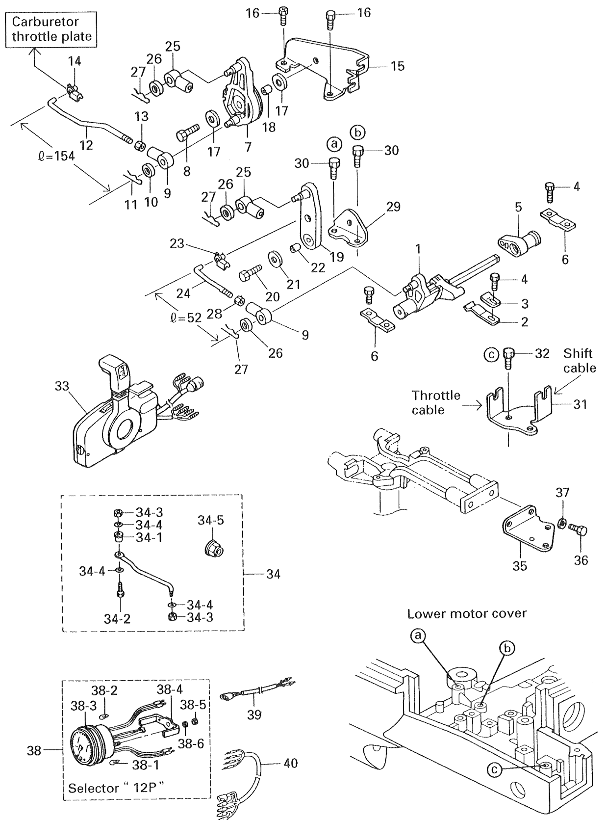
シフト SHIFT Fig. 17
