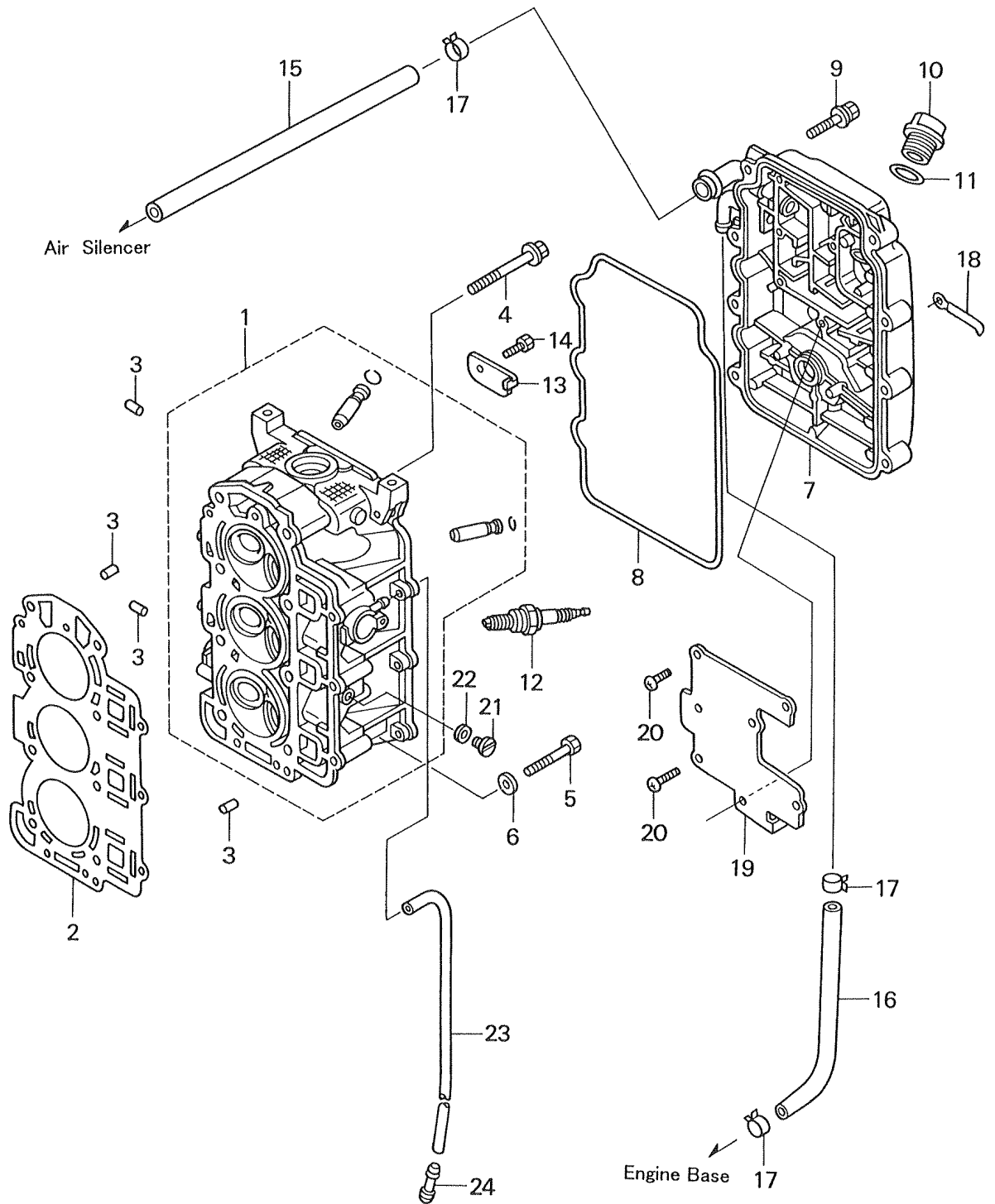
シリンダヘッド Fig. 1 CYLINDER HEAD
