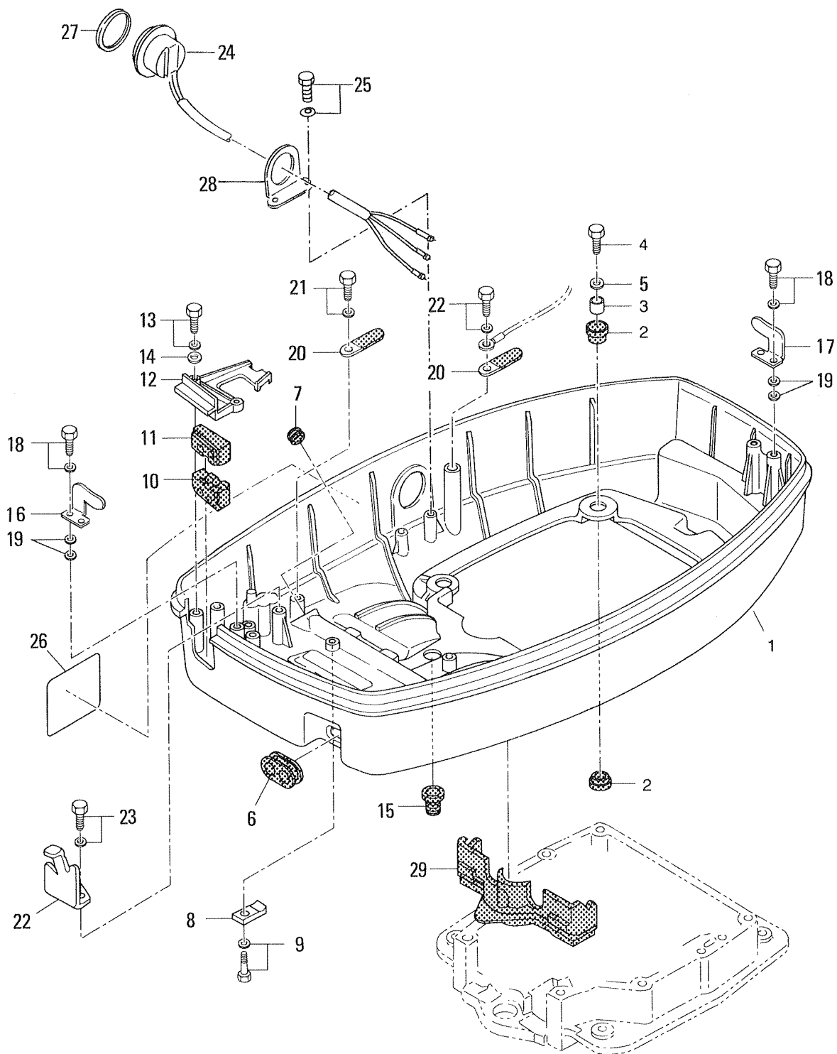
ロウモータカバー Fig. 19 LOWER MOTOR COVER
