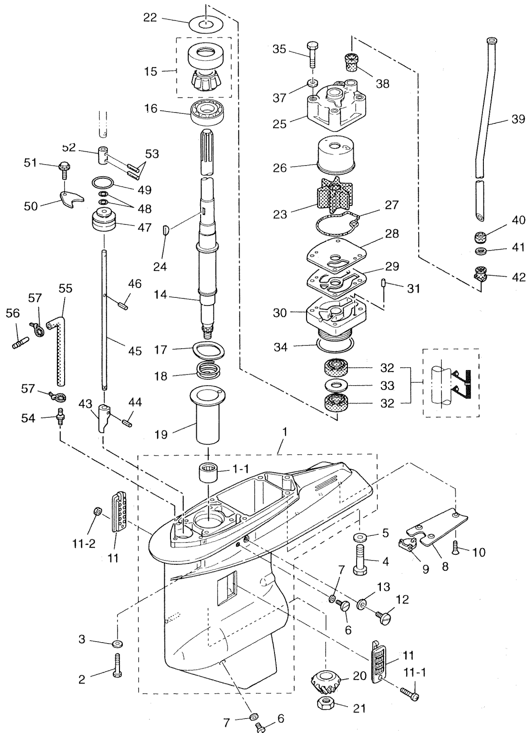
ギヤケース (ドライブシャフト) 2 Fig. 15 GEAR CASE (DRIVE SHAFT) 2
