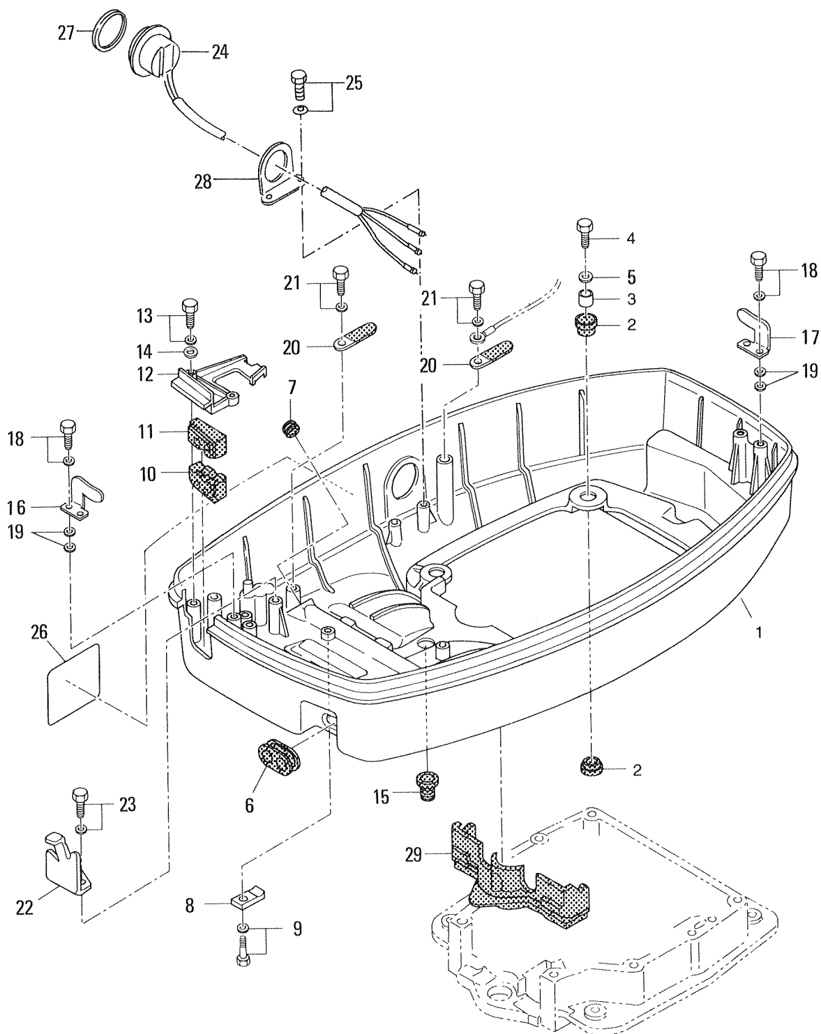
ロワモータカバー Fig. 20 LOWER MOTOR COVER
