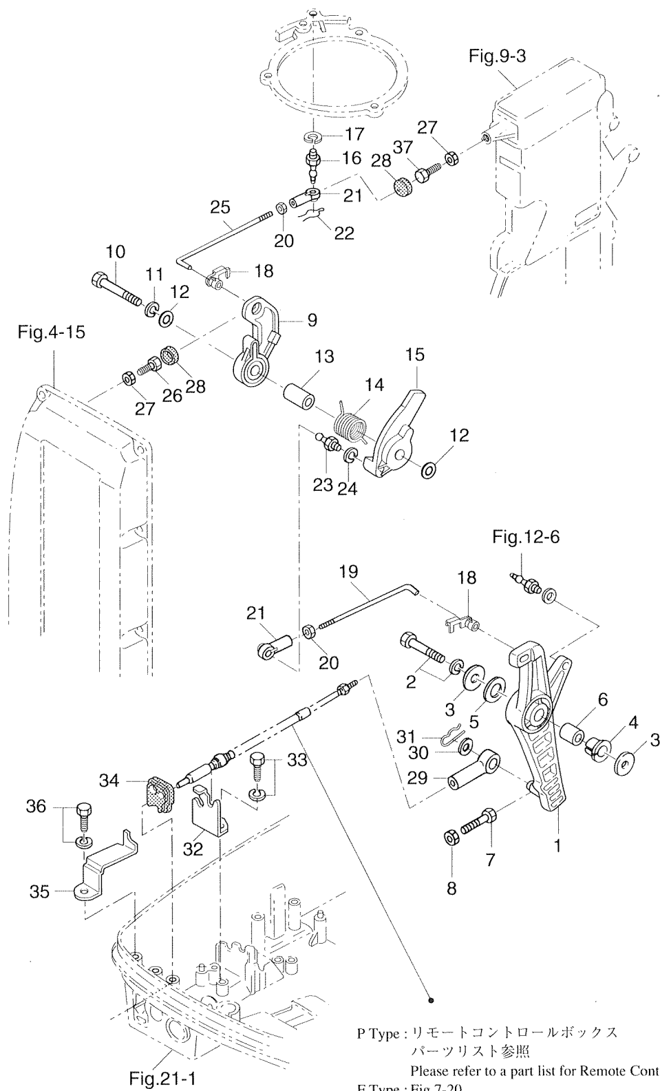
Fig. 6 THROTTLE (cont.)
