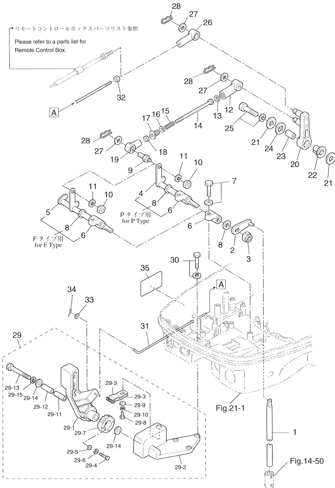
Fig. 16 SHIFT
