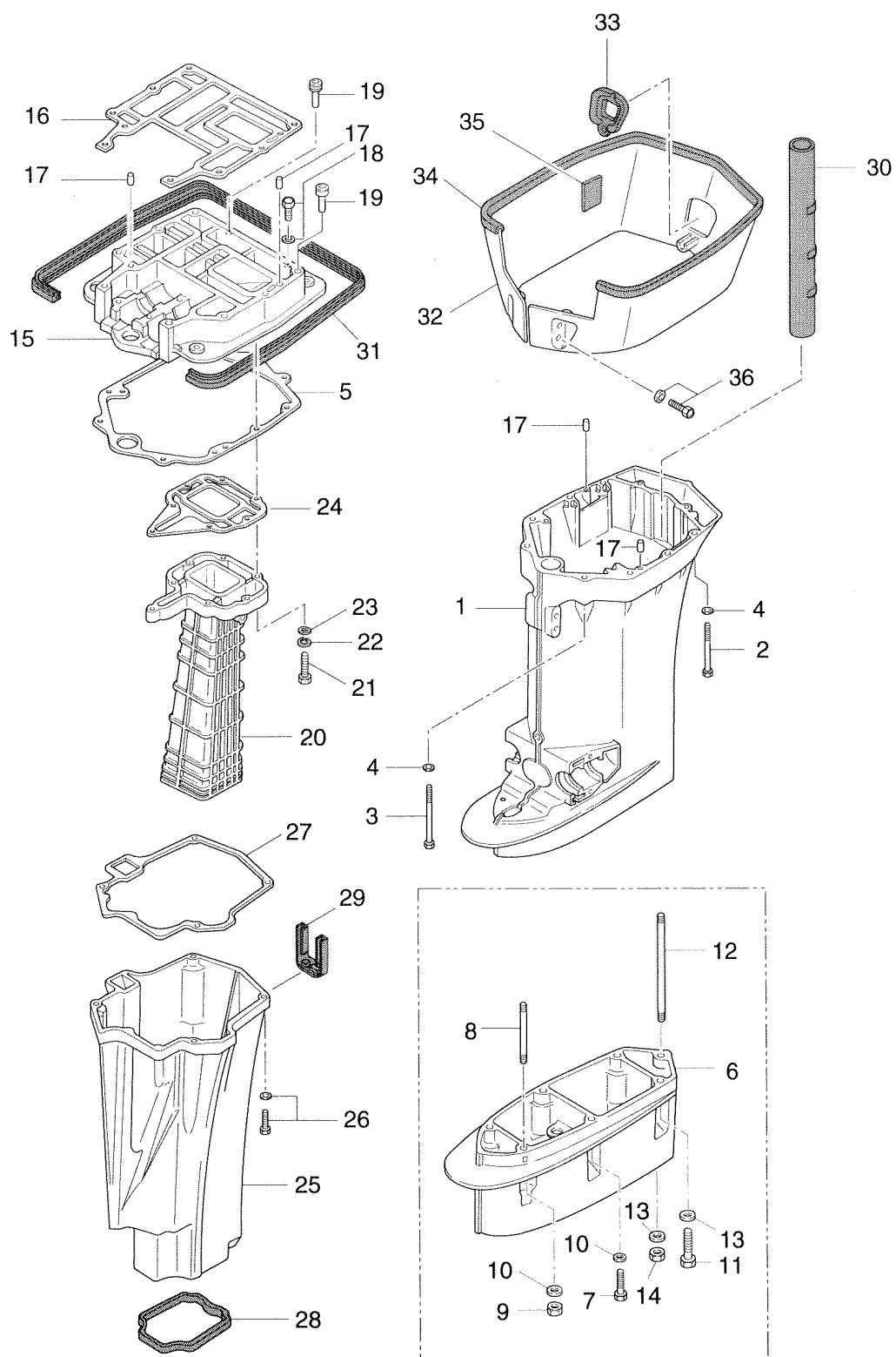
ドライブシャフトハウジング Fig. 13 DRIVE SHAFT HOUSING (cont.)
