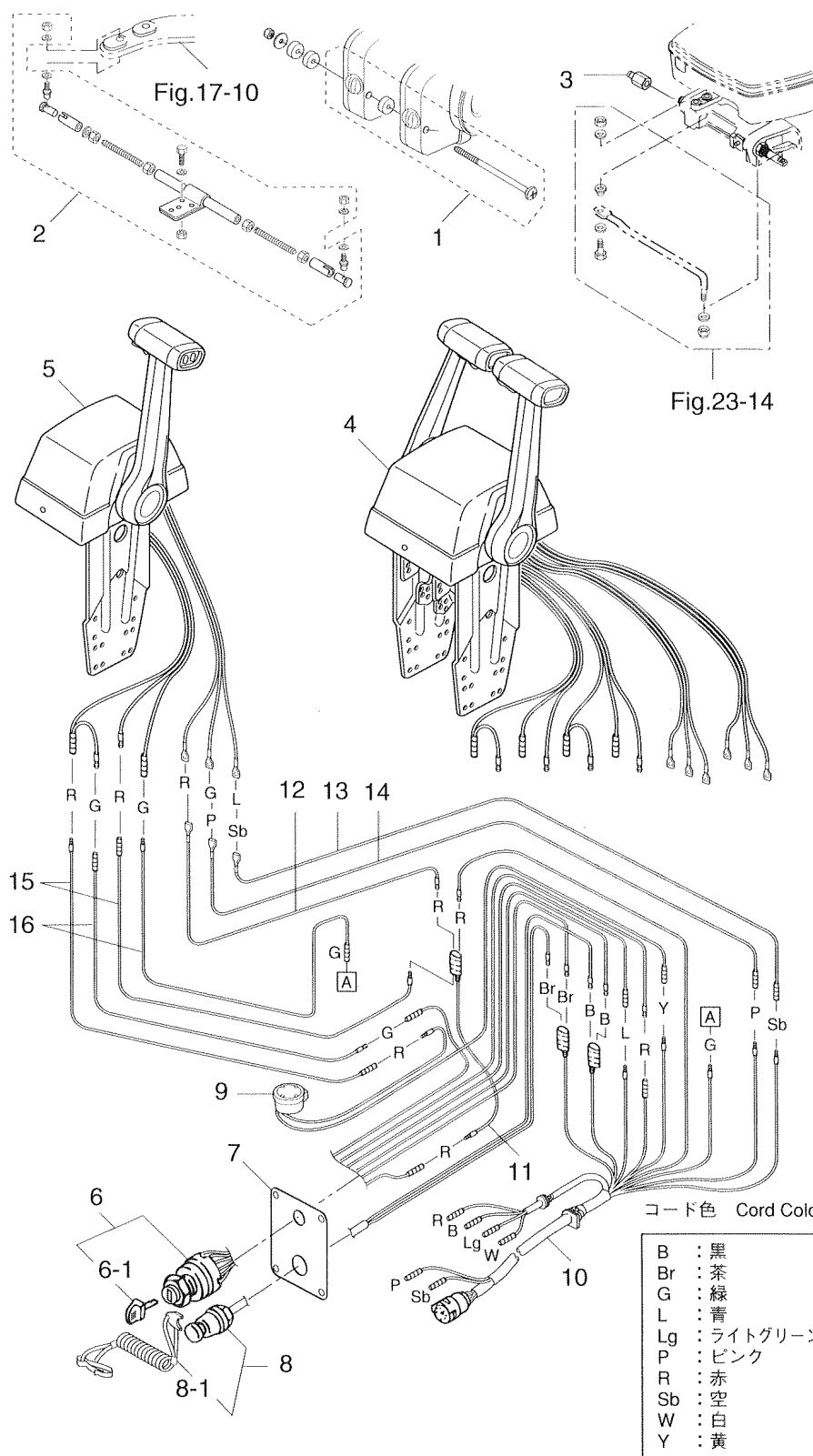
Fig. 25 OPTIONAL PARTS (2)
