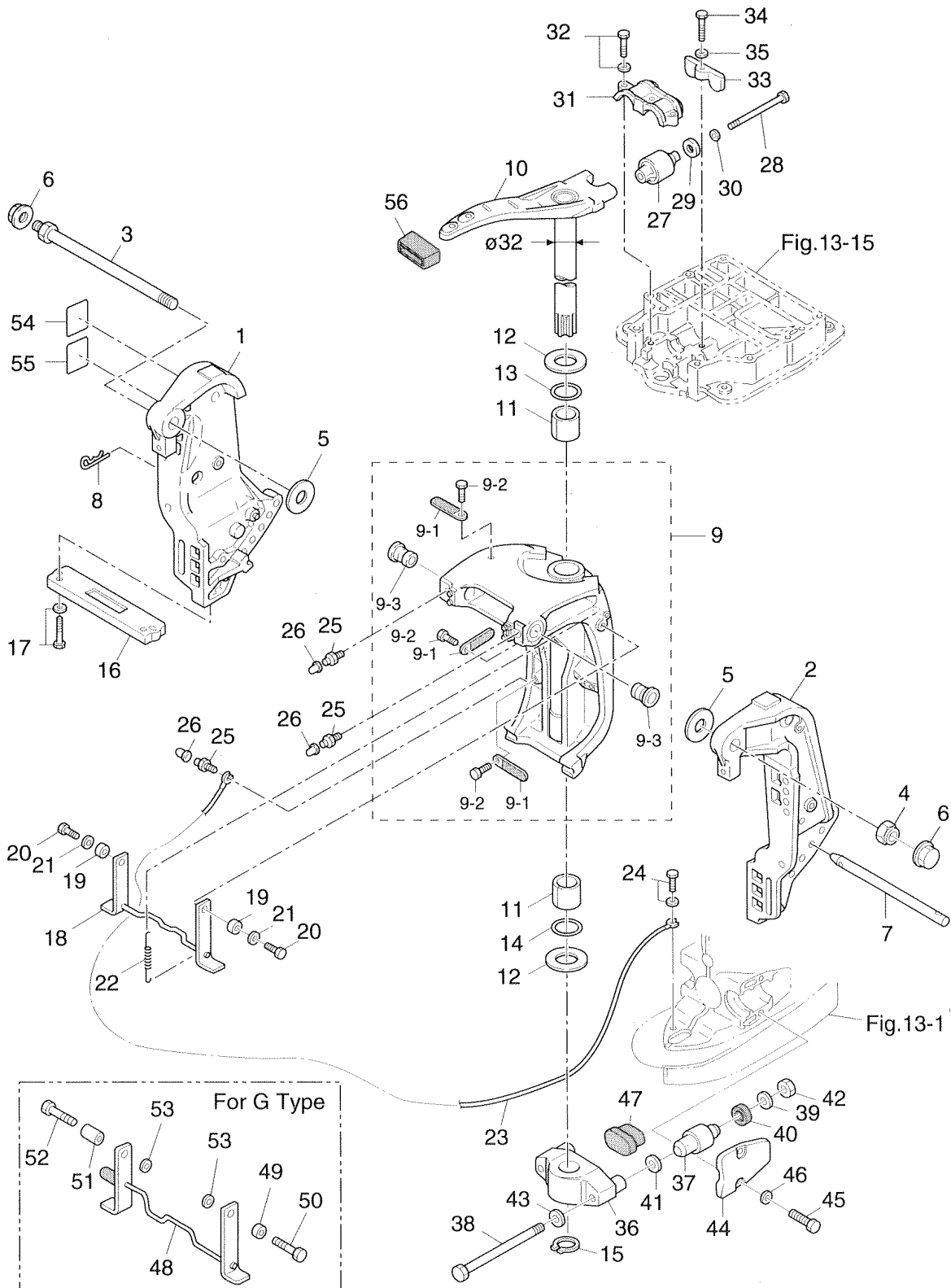
Fig. 17 BRACKET (cont.)
