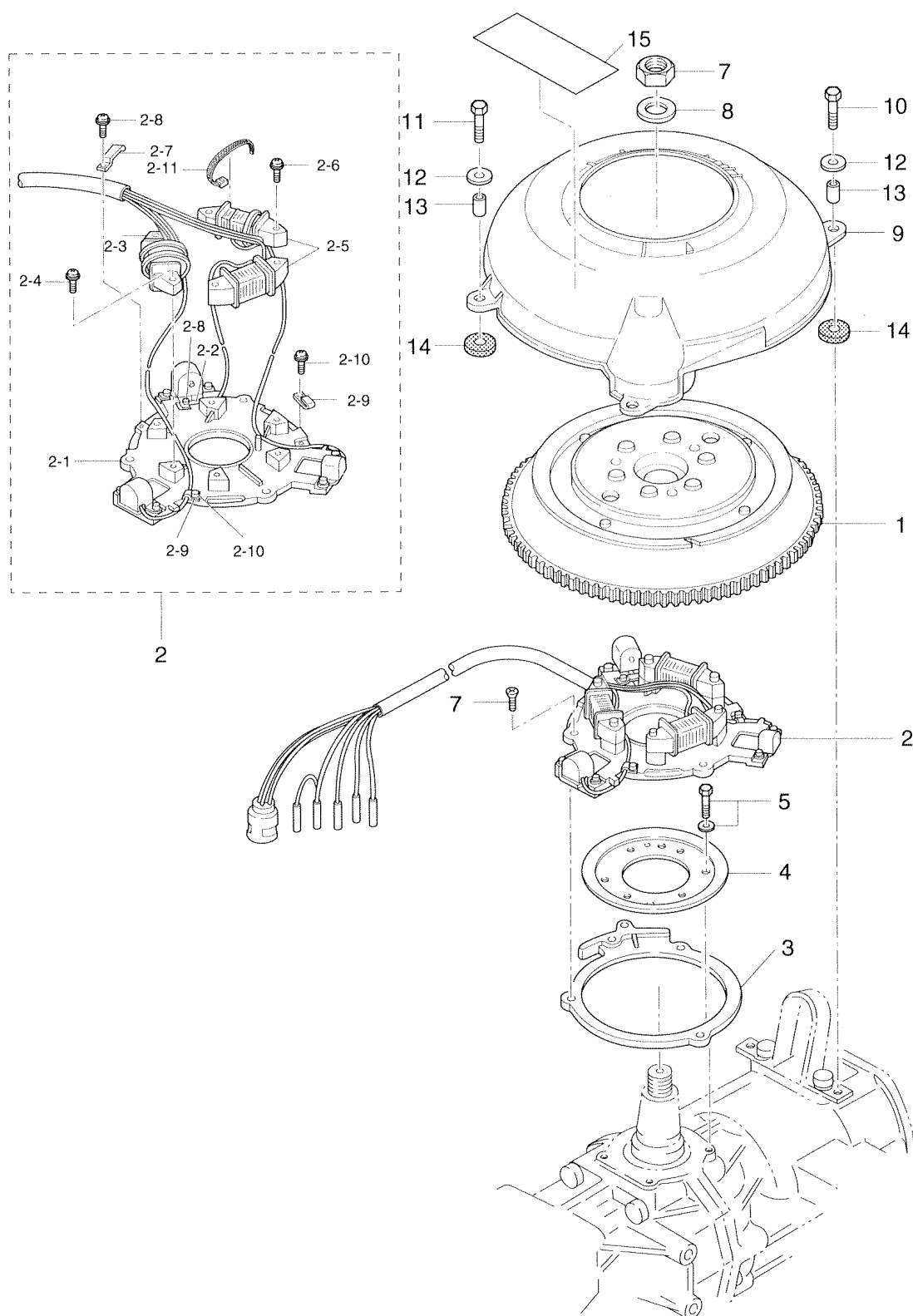
Fig. 8 MAGNETO
