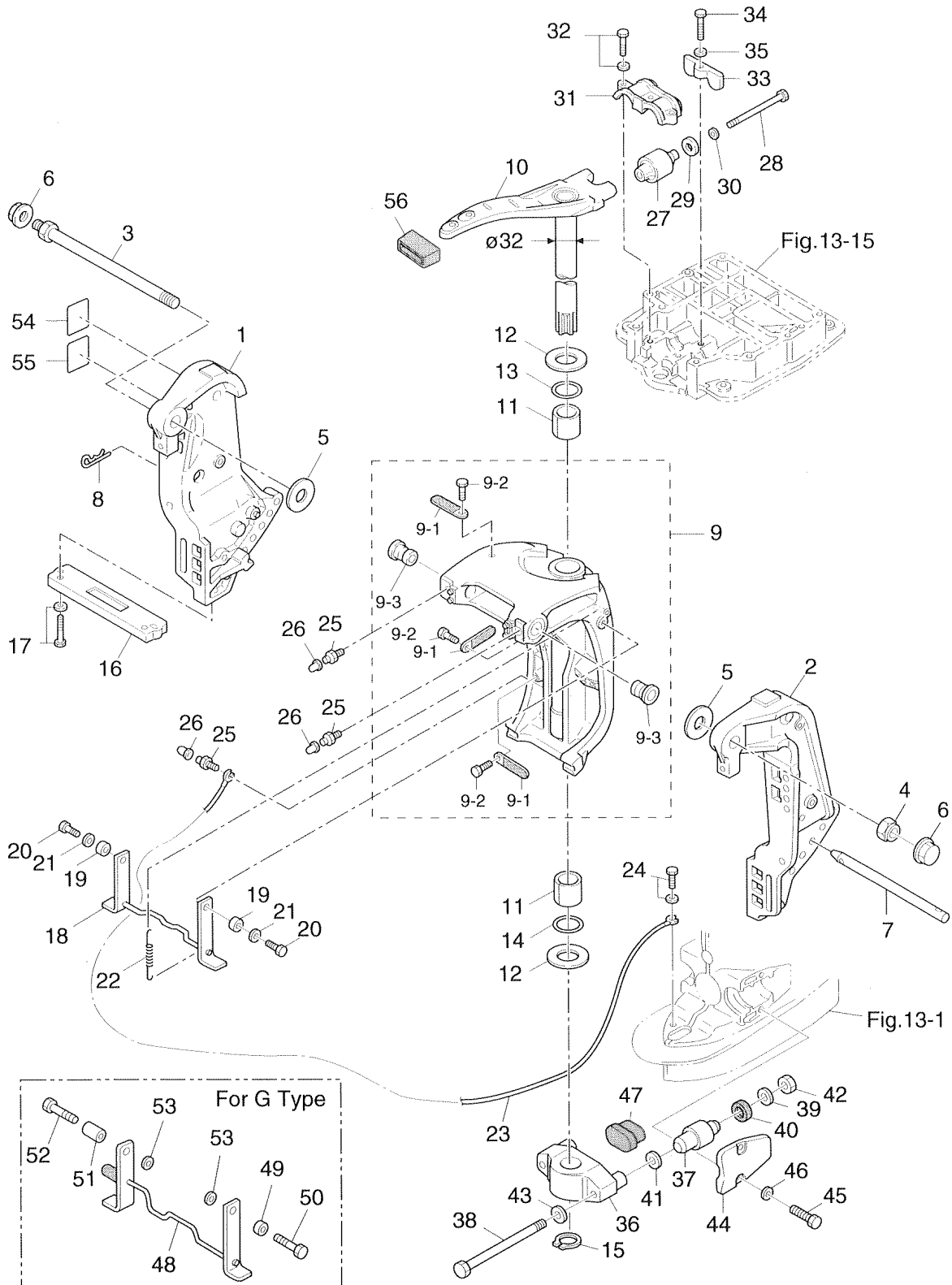
Fig. 17 BRACKET (cont.)
