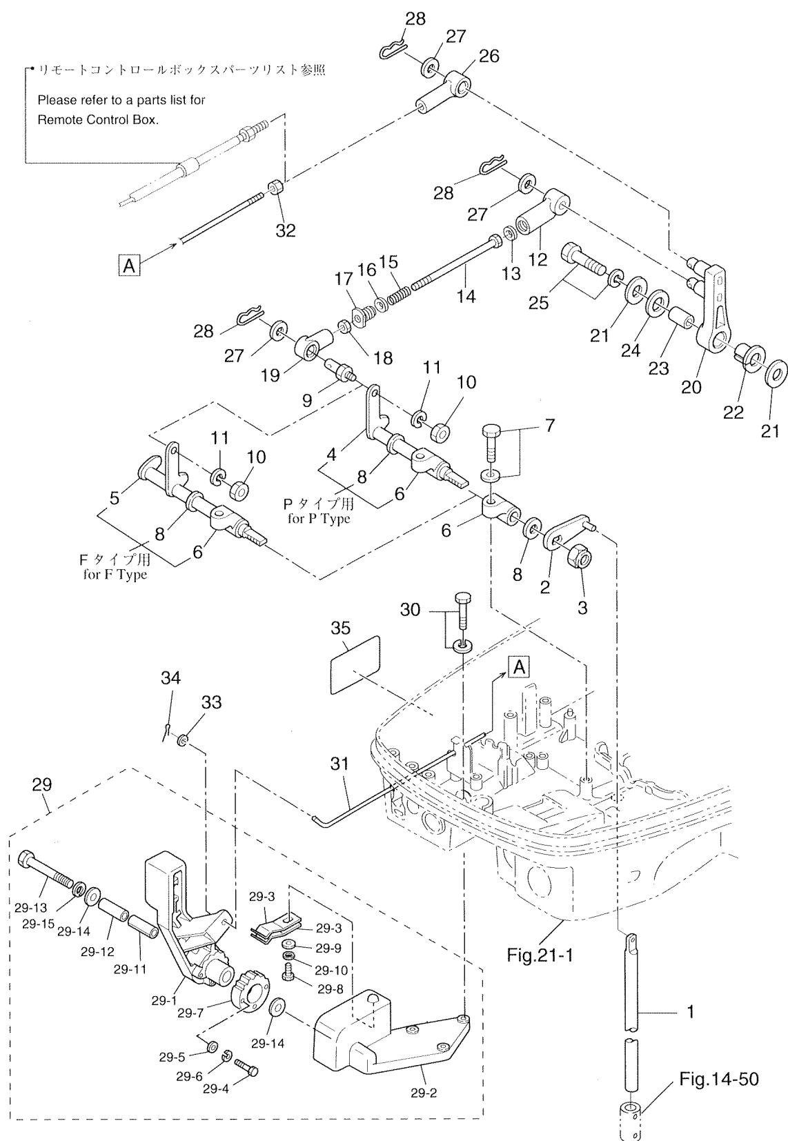
Fig. 16 SHIFT (cont.)
