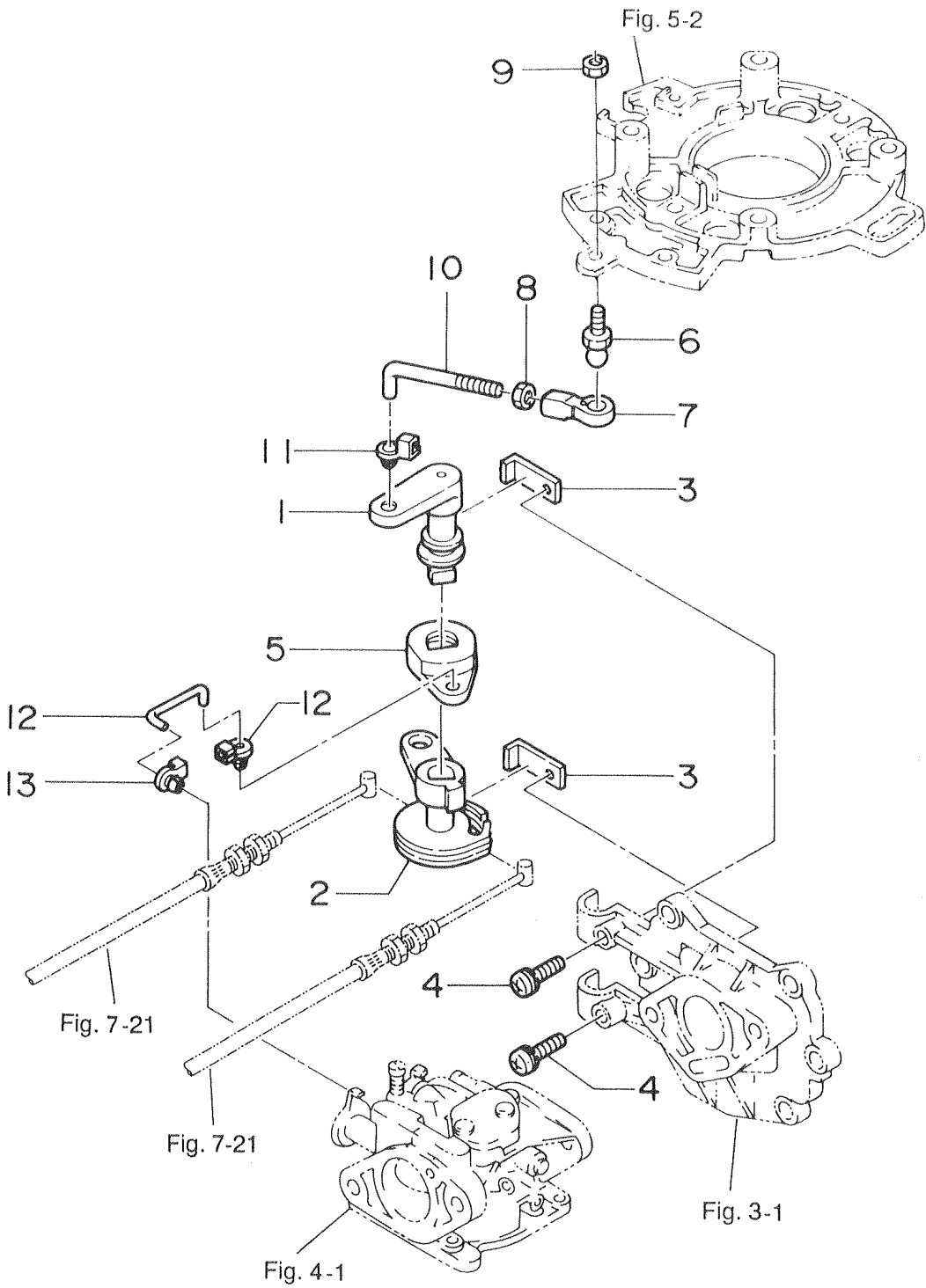
スロットルメカニズム THROTTLE MECHANISM
