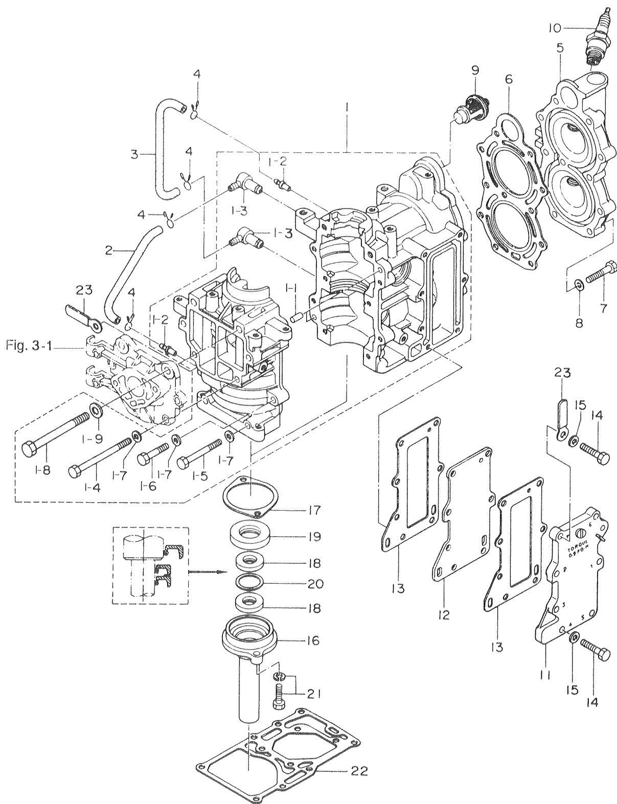
シリンダ・クランクケースアッシー CYLINDER · CRANK CASE ASS'Y
